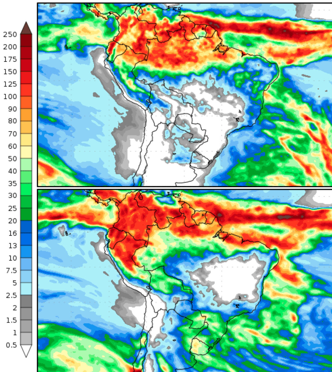
Figura 1. Precipitação acumulada prevista entre os dias 11 a 19 de maio (imagem superior) e 19 a 27 de maio de 2023 (imagem inferior). Fonte: COLA (Center for Ocean-Land-Atmosphere-Studies).
